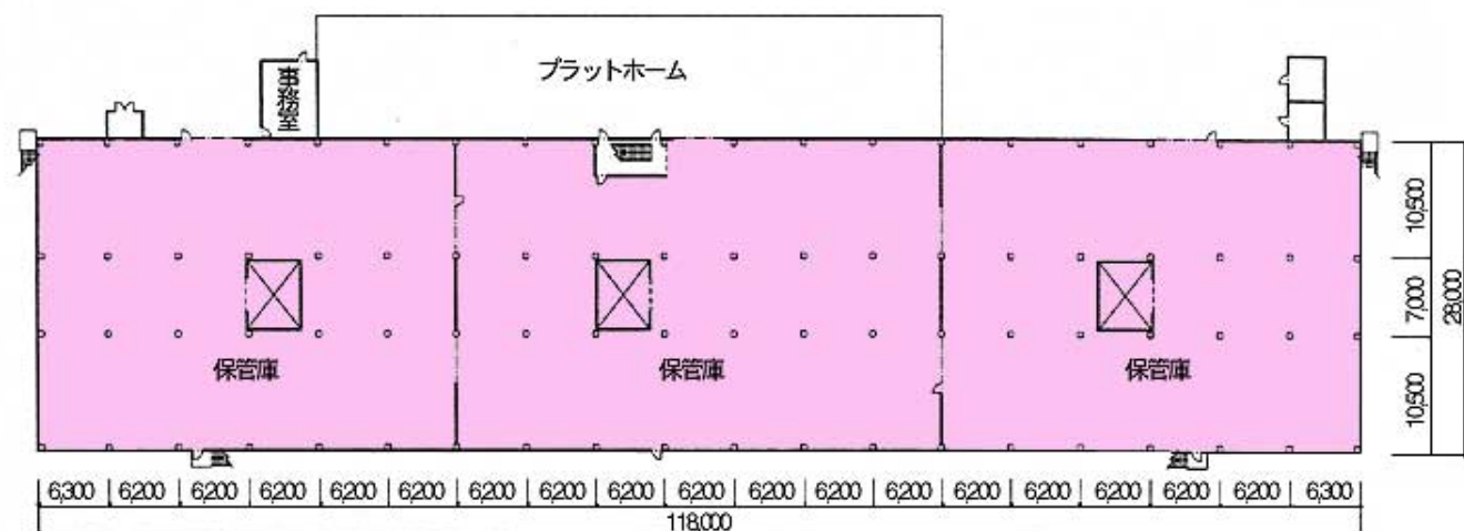
1 F 平面図
