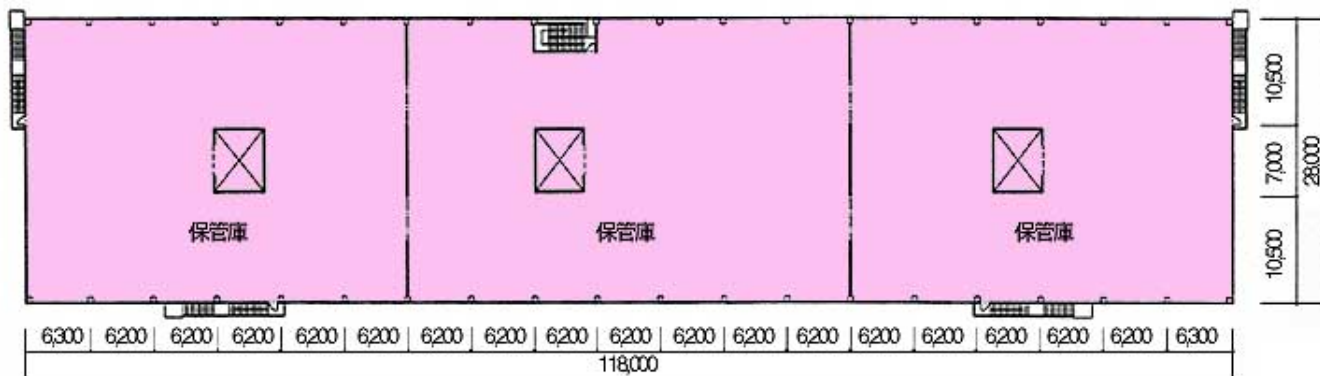
3 F 平面図
