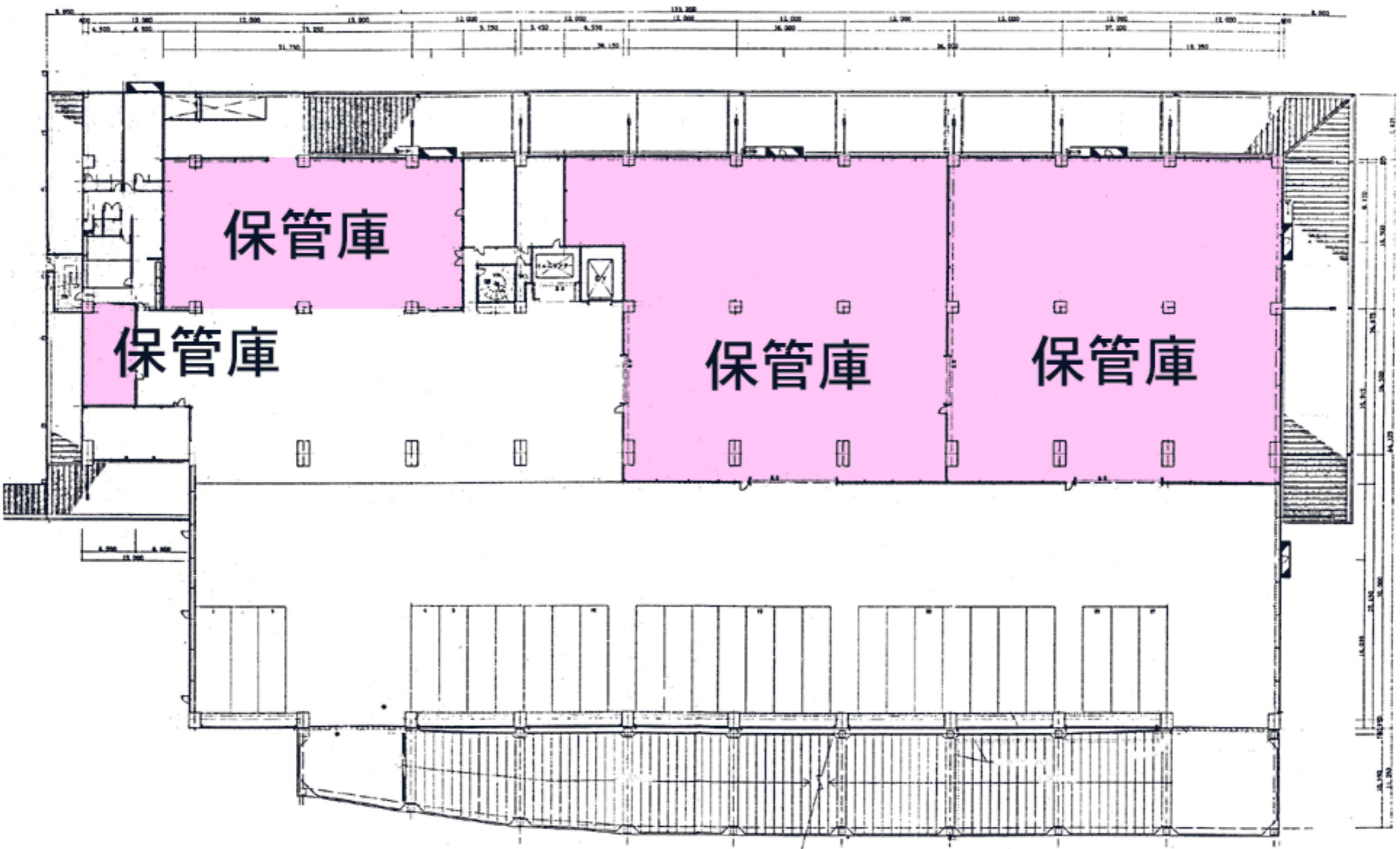
3F 平面図
