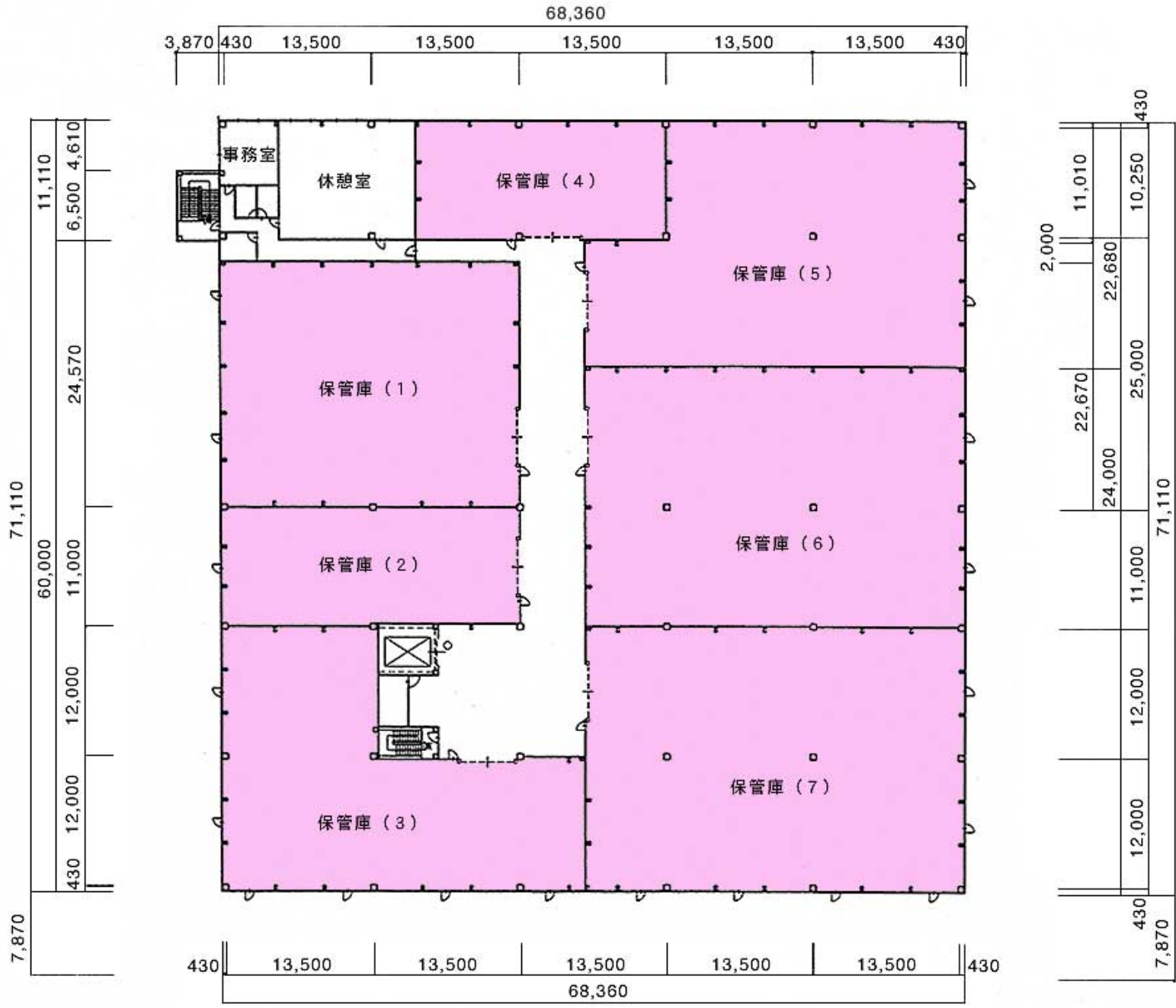
2F平面図
