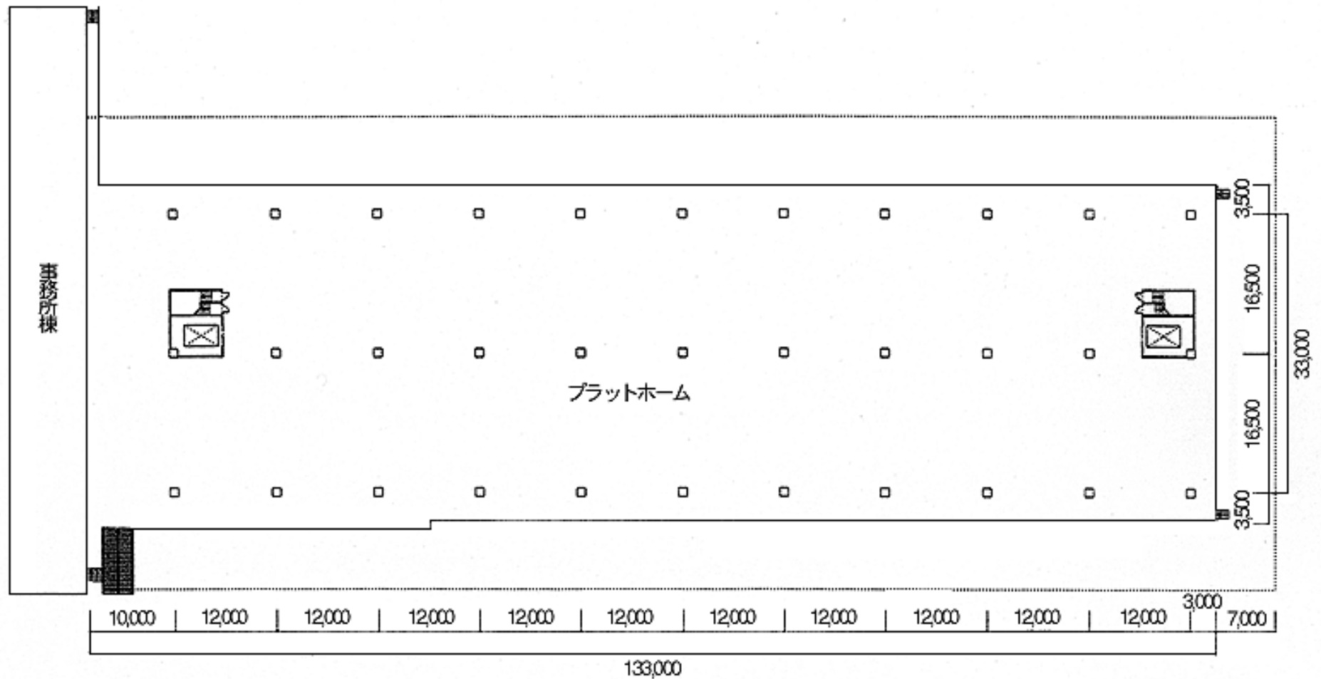
1F平面図
